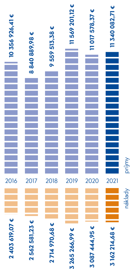
Vývoj príjmov a nákladov SOZA 2016-2021
